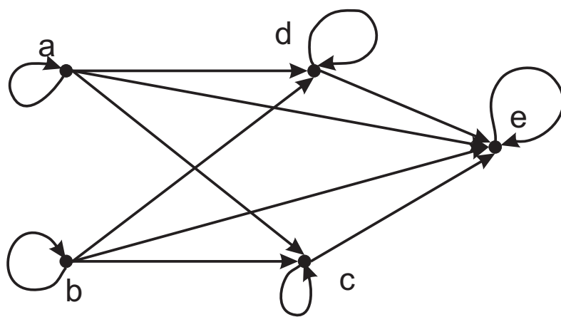
ациклический граф
